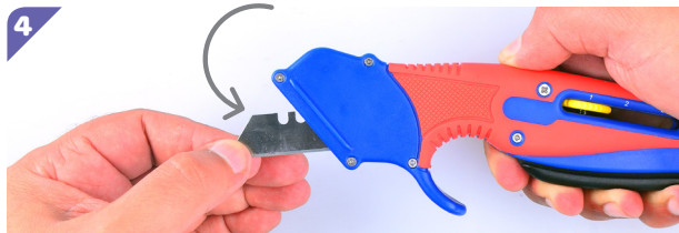
Continuez à garder la gâchette appuyée pendant que vous introduisez la nouvelle lame LSP 072 jusqu'à ce que la lame soit en butée.
